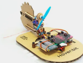
micro:bit hovercraft SKU: 222-9374 MPN: Hover:bit 2.0 Single
